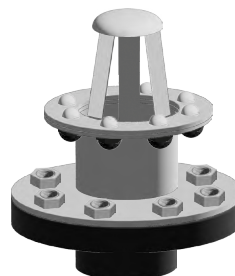
Vidange par le fond Bloc bride avec antivortex inox boulonné Collet bride PVC-P DN110 (raccordement tuyauterie enterrée à coller)
