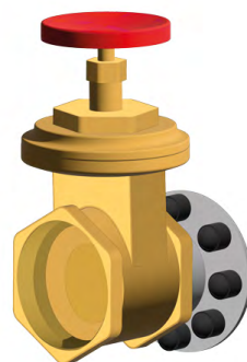
Remplissage/Vidange sur le flanc Vanne guillotine laiton DN100 Bride inox
